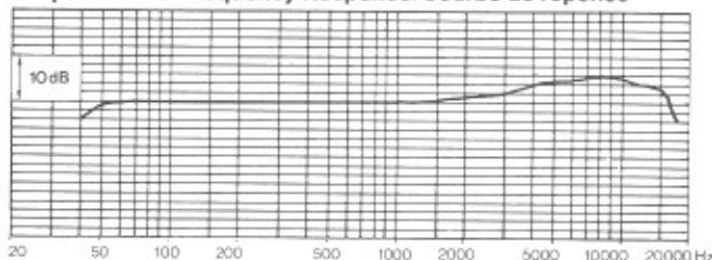
Frequenzkurve/Frequency Response/Courbe de réponse
